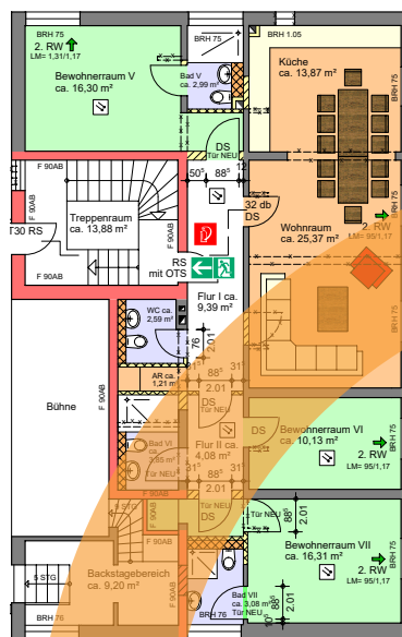
CVJM HOMEBASE 1. Etage mit 3 Zimmern und Gemeinschaftsraum
